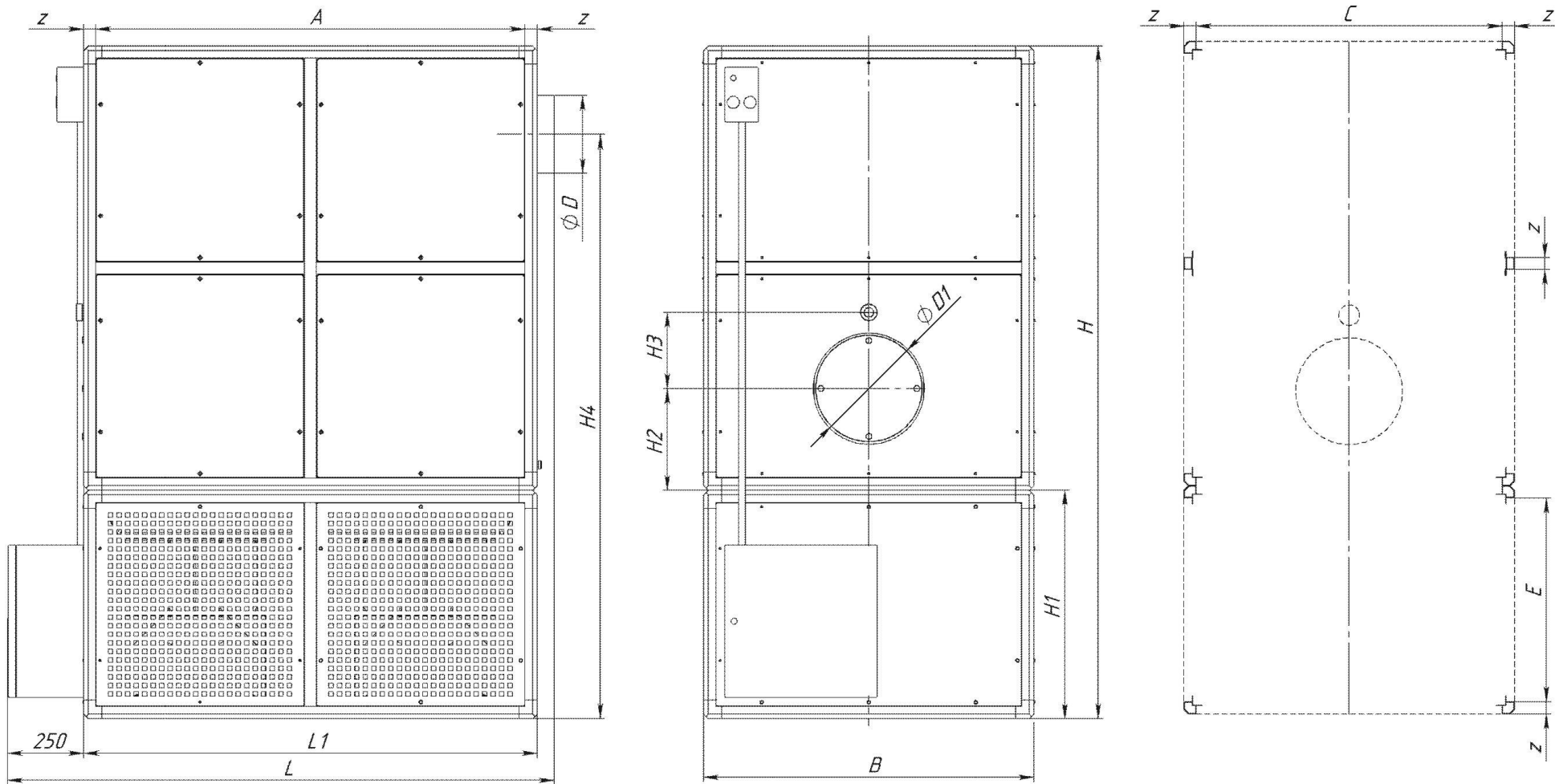
Габаритные размеры воздухонагревателя TITAN Air VSV
