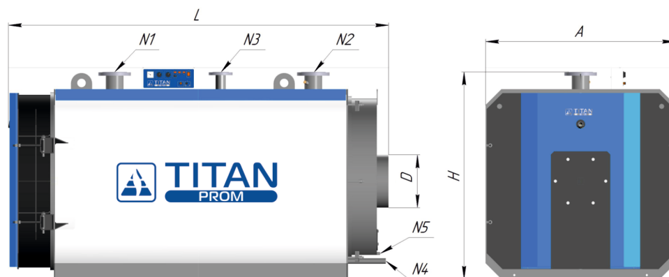
Технические характеристики и размеры котлов TITAN PROM
